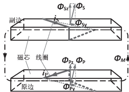
(d) 原边正绕，副边反绕翻转变压器磁通量分布
