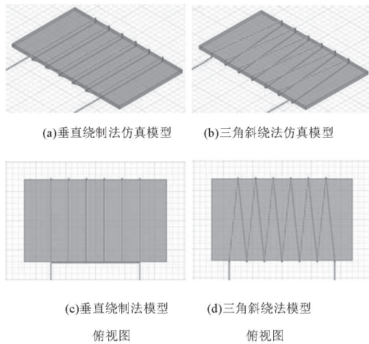
图 2 垂直绕制法和三角斜绕法 3D 有限元仿真模型
