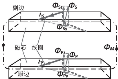
(a) 原边正绕，副边正绕变压器磁通量分布
