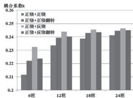
图 8 不同匝数时，绕制方法对耦合系数影响的仿真结果
