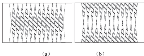
图 6 (a) 原边正绕，副边正绕翻转 (b) 原边正绕，副边反绕翻转时垂直方向耦合情况俯视图
