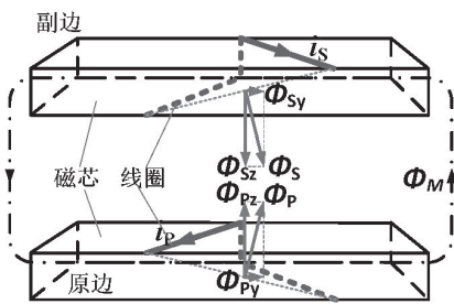
(b) 原边正绕，副边反绕变压器磁通量分布
