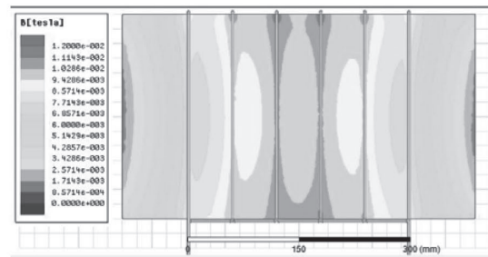
(a) 垂直绕制法模型磁芯内部磁感应强度分布图
