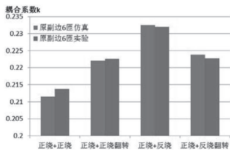
图 7 原边副边各 6 匝四种线圈绕制组合仿真结果与实验结果
