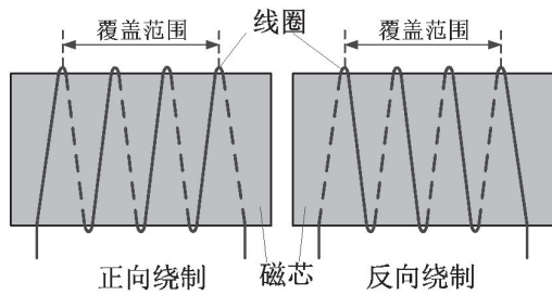
图 4 正绕法、反绕法绕制方法示意图
