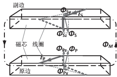
(c) 原边正绕，副边正绕翻转变压器磁通量分布
